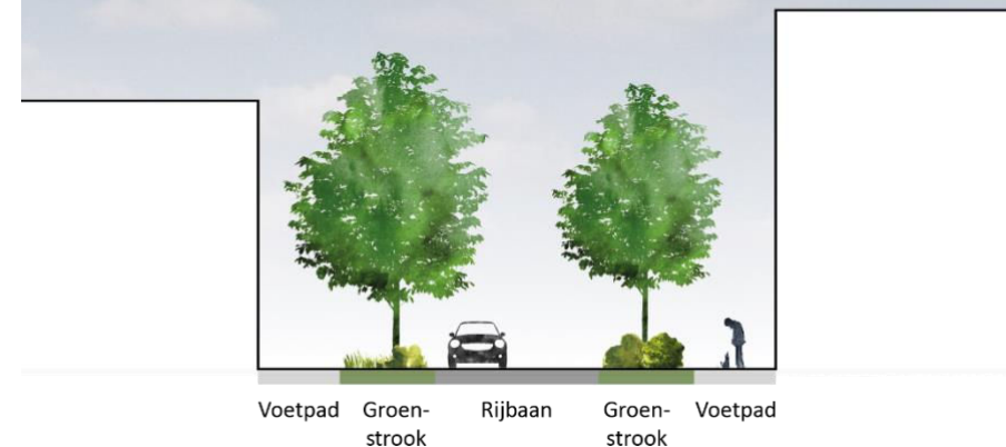
Figuur 4: Voorbeeld profiel voor een wijkontsluitingsweg. De benodigde breedte van het profiel is ook afhankelijk van de hoogte van de omliggende bebouwing.
